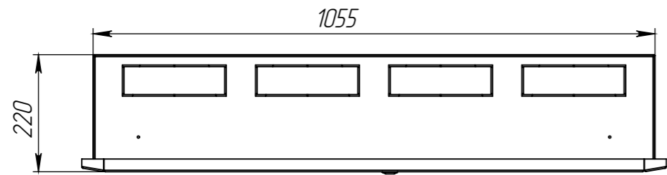
A-A (1 : 10)
