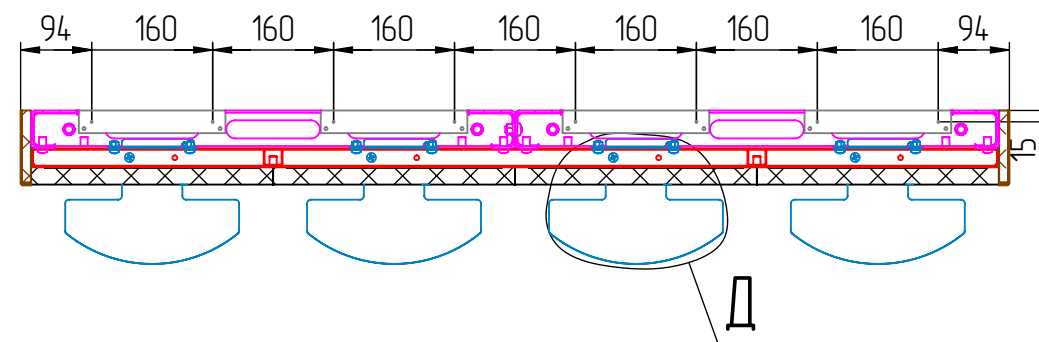
A2-A2 (1:10)
