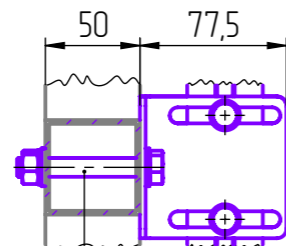
Болт M10x70 DIN 933 Гайка M10 DIN 934 Шайба 10 DIN 125 Шайба 10 DIN 7980
