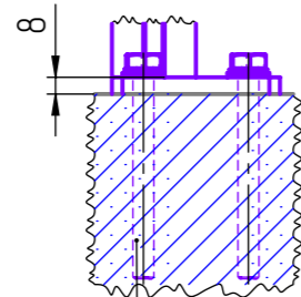
Анкер мунд Hilti HSA-F M10x83
