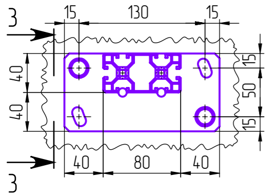
Узел крепления к полу. M1:4
