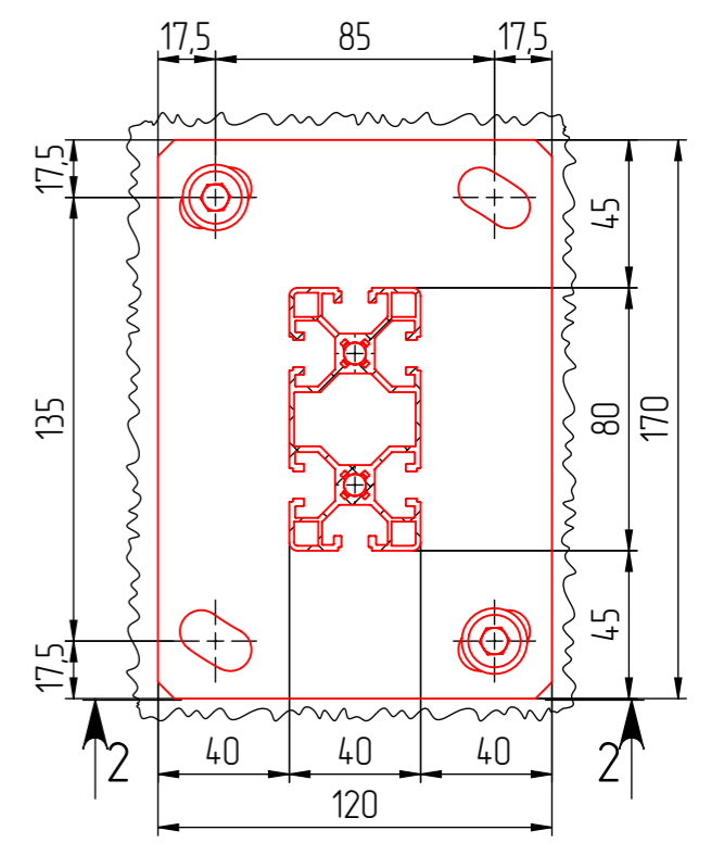
Узел крепления к полу
