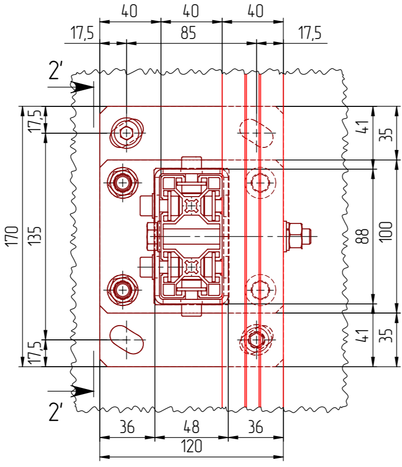
Узел крепления к стене
