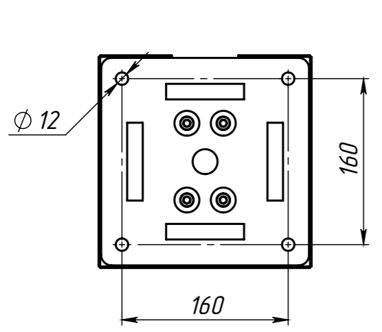
Б-Б (1 : 5)
